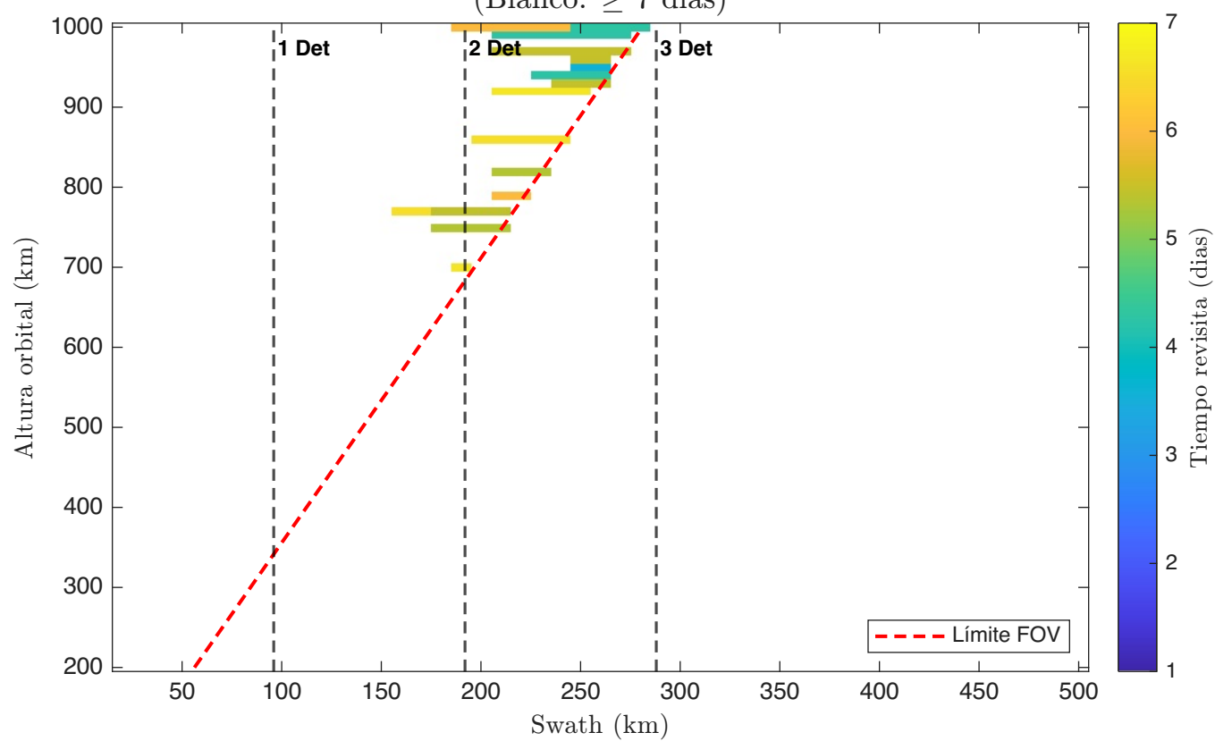
Tiempo Revisita - 2 Satellite(s); 2 Telescopio(s): TMA; Detector 1 (Blanco: \geq 7 días)
